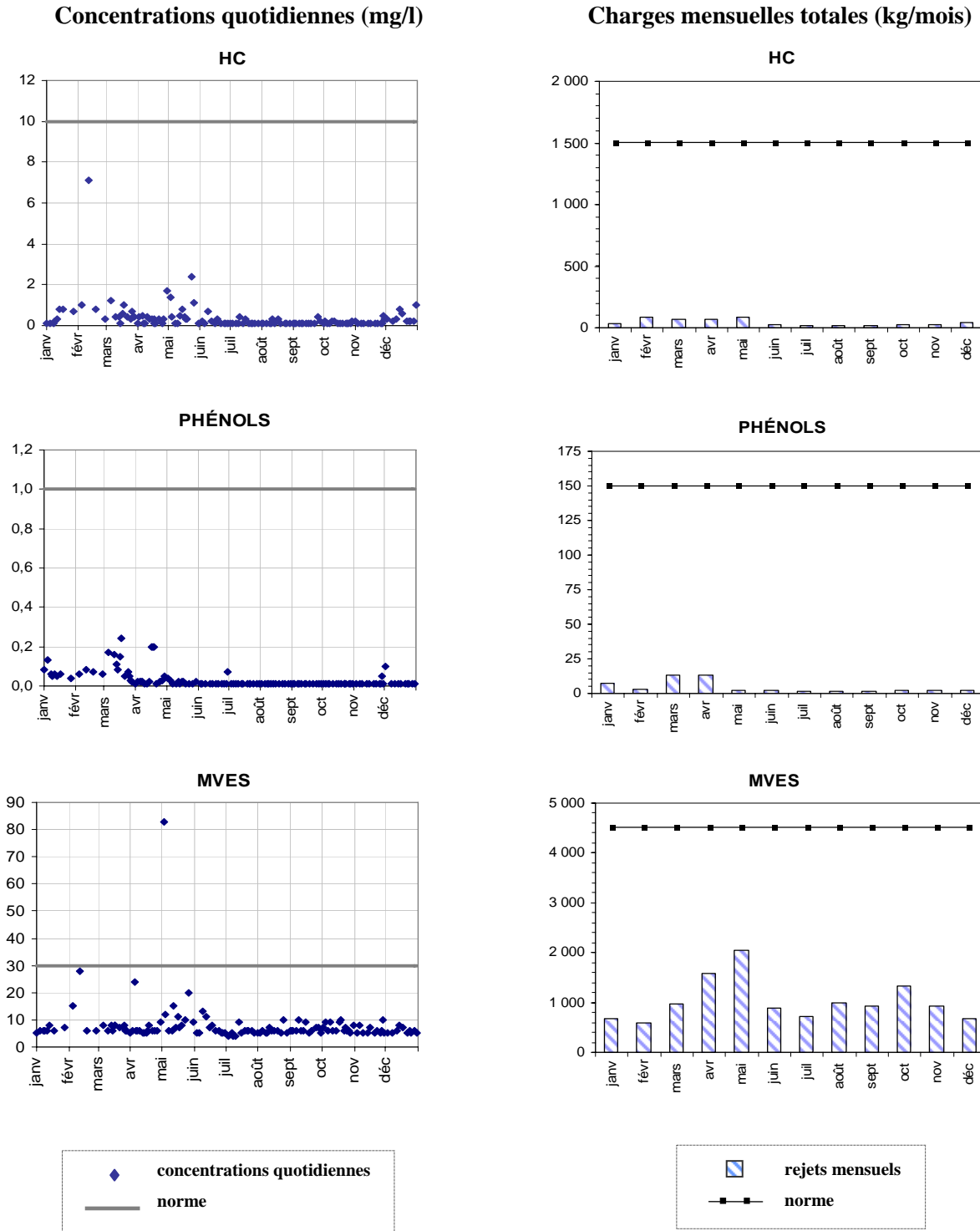
Figure B - 3 Concentrations quotidiennes et charges mensuelles totales dans l'effluent d'eaux pluviales de Pétro-Canada en 2007 en comparaison des normes
