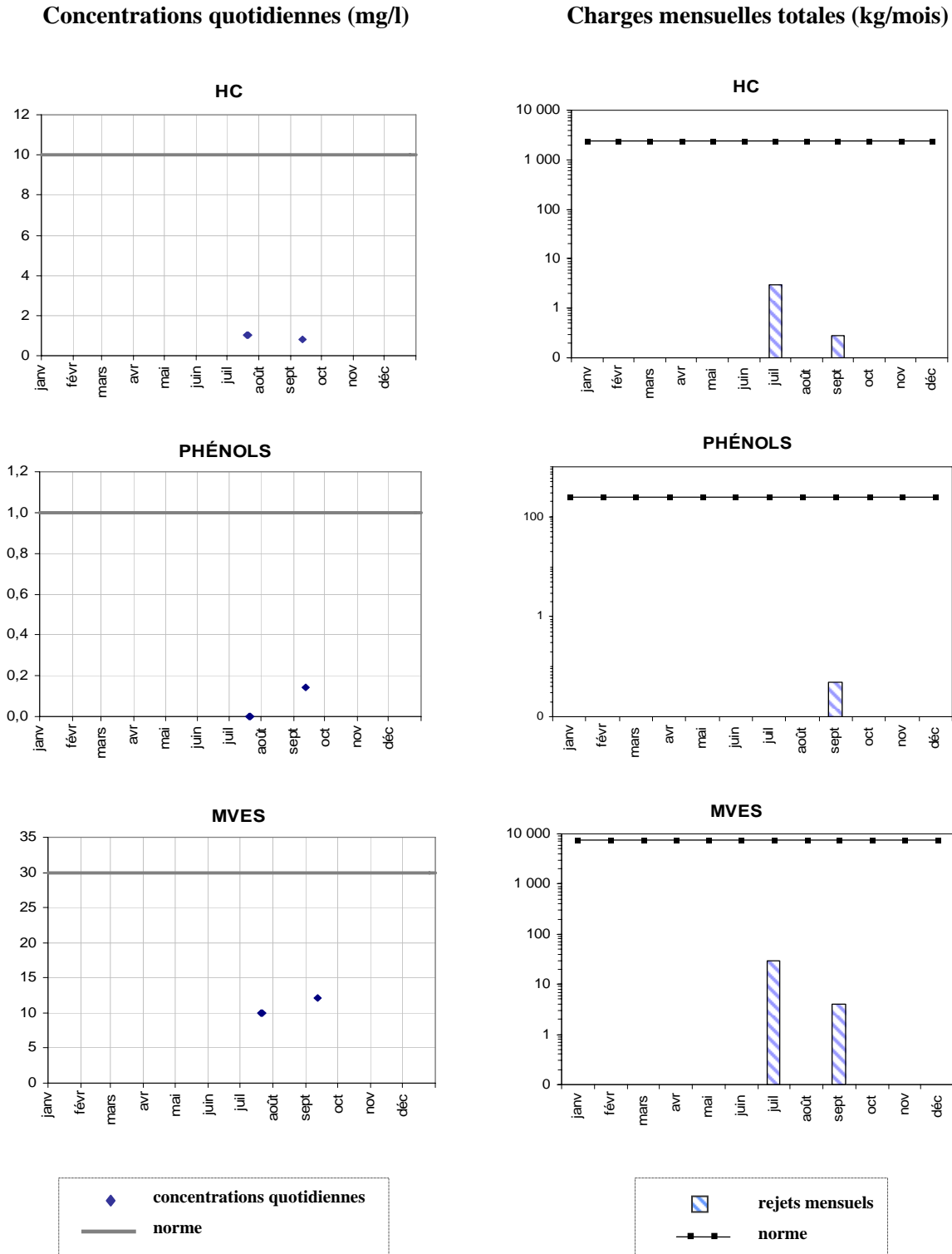
Figure B - 9 Concentrations quotidiennes et charges mensuelles totales dans l'effluent d'eaux pluviales d'Ultramar en 2007 en comparaison des normes
